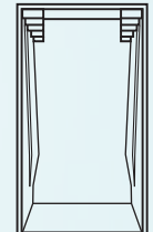
TILOS L 7,00 m x l 3,50 m Prof. 1,50 m Fond plat
