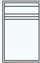
THILIA L 6,30 m x l 3,40 m Prof. 1,50 m Fond plat
